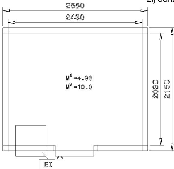
Zij aanzicht
